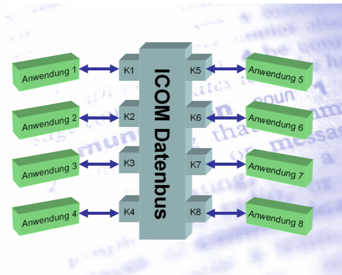
Abbildung. 2: Nur über ein EAI-Werkzeug wie ICOM bleiben Kommunikationsnetze beherrschbar
